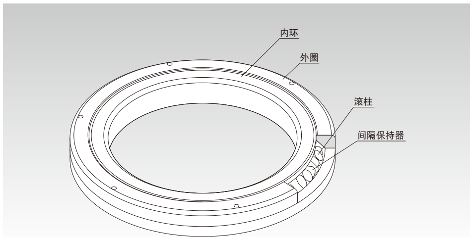
图1 交叉滚柱轴环RB型的结构
