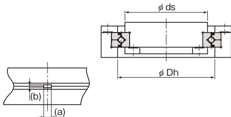
润滑孔的详细视图
